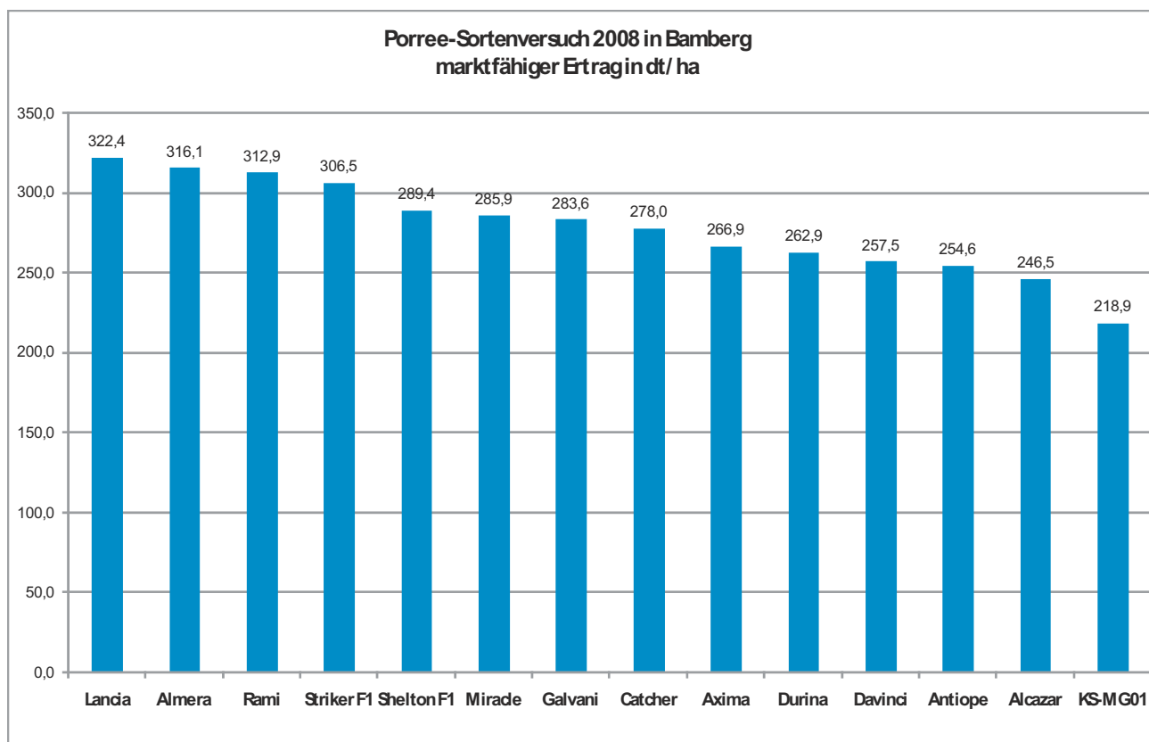
Abb. 1: marktfähiger Ertrag
