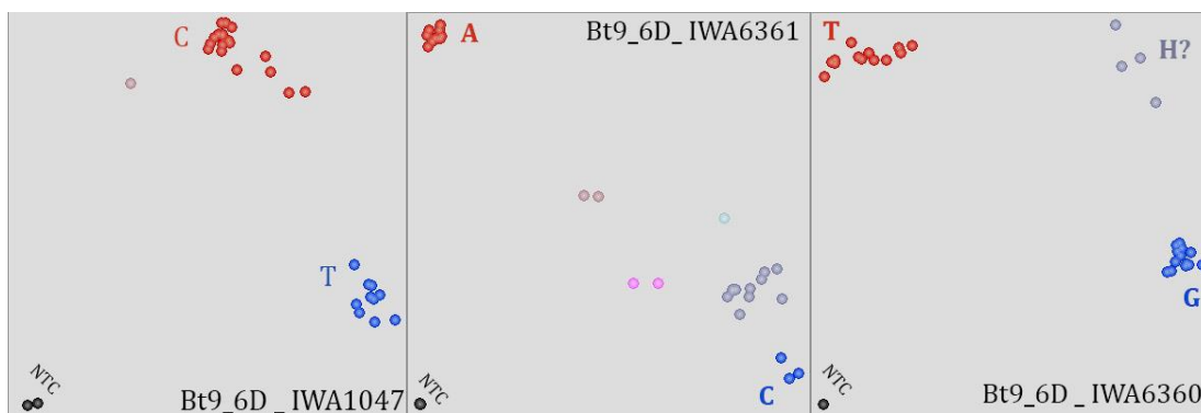
Figura 2. Analize KASP pentru gena Bt9
